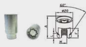
CONICAL NUT + CYLINDRICAL 60° DADO CONICO + CILINDRICO 60°
