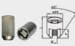
NUT 60° DADO 60°
